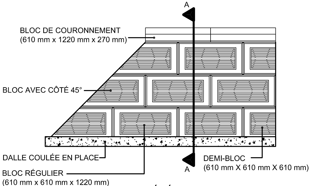
ÉLÉVATION
